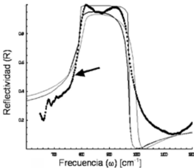
Fig. 5. Espectros R-FTIR experimental (con flecha) y calculados para una muestra 3C-SiC/Si.
