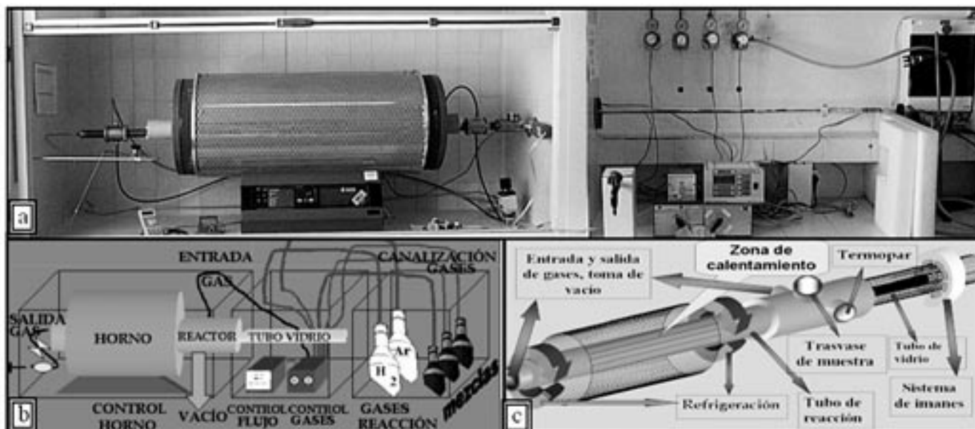
Fig. 1. Fotografía (a) y esquema (b) del sistema de carburización. Esquema del reactor de carburización (c).
